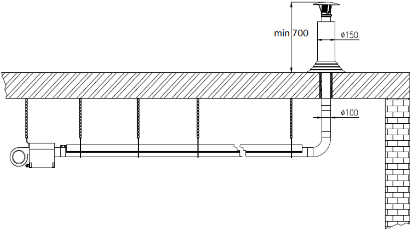
Şekil 6.7.2 Baca bağlantı örnekleri
