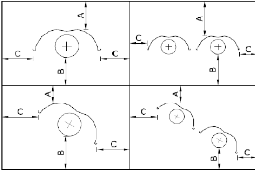
Şekil 6.2.1 Yanıcı maddelere uzaklık
