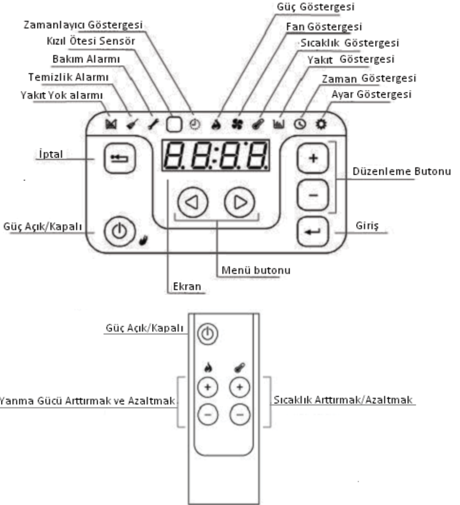
řekil 11: Tuř takımı(Klavye) ve uzaktan kumanda tanımlamaları
