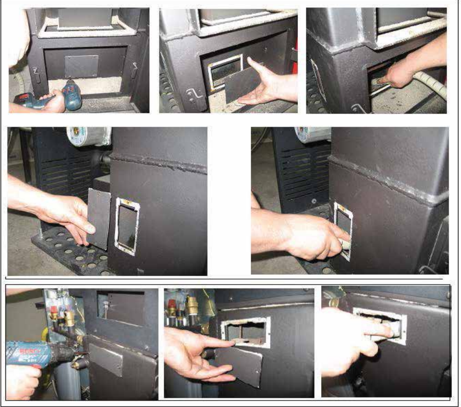
Şekil 20: Yanma odası alt, yan ve üst arka haznelerin temizlenmesi
