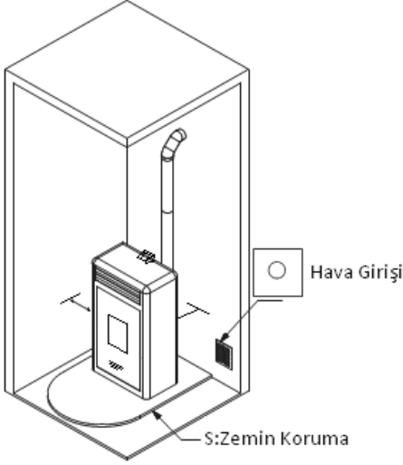
Şekil 1: Harici hava girişi
